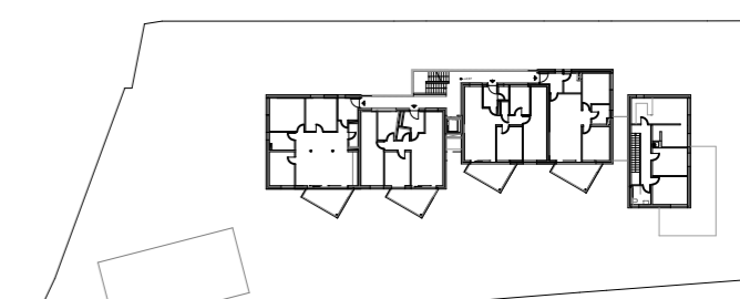
1. OBERGESCHOSS
