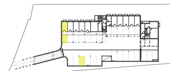
UNTERGESCHOSS
