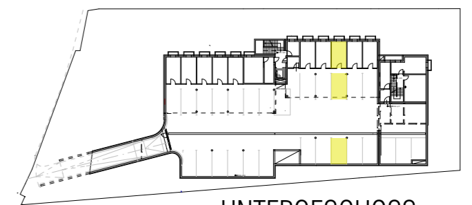
UNTERGESCHOSS
